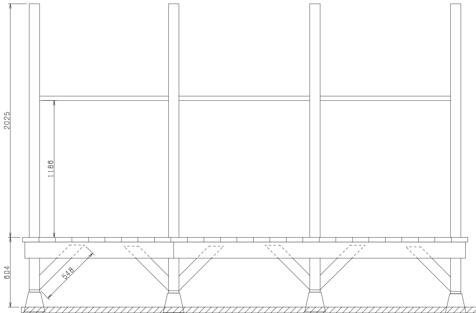
立面图(前)
